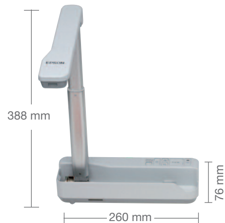
Wymiary (rozłożony)
